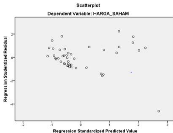
Gambar 5. Hasil Pengujian Heteroskedastisitas
