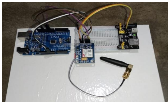
Gambar 15. SIM 800L
