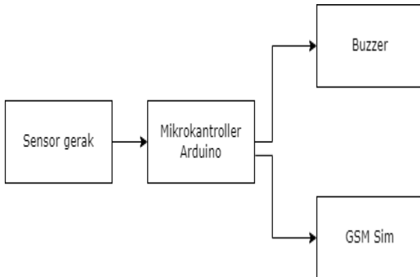
Gambar 9. Blok Diagram Sistem
