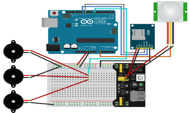
Gambar 11. Perancangan Alat Sensor Keamanan Ruangan
