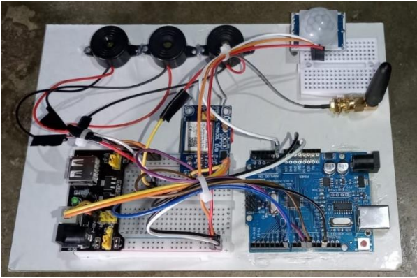
Gambar 18. Alat Sensor
