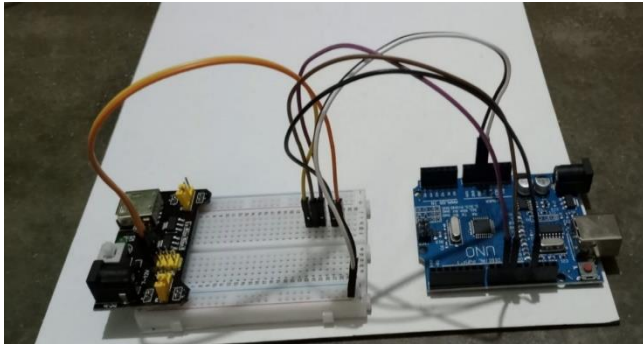
Gambar 14. Arduino dan Power Supply
