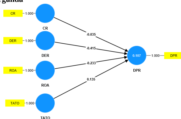
Gambar 2. Analisis Regresi Linear Berganda
